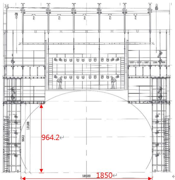
GP 鏡框板打開正視圖(單位：cm)
