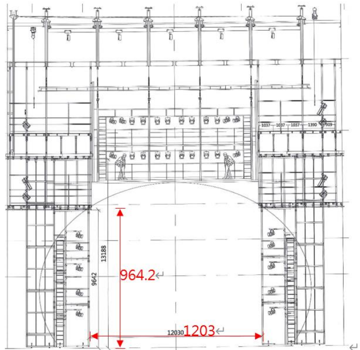
GP 鏡框板合攏正視圖(單位：cm)
