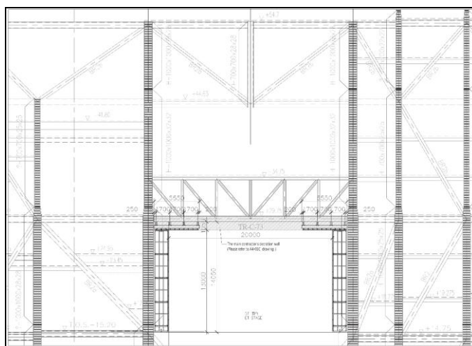
GT 鏡框板打開正視圖
